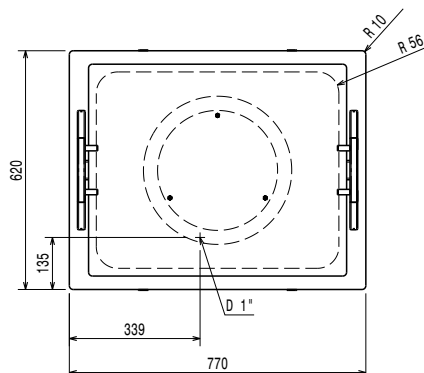
Boven aanzicht
